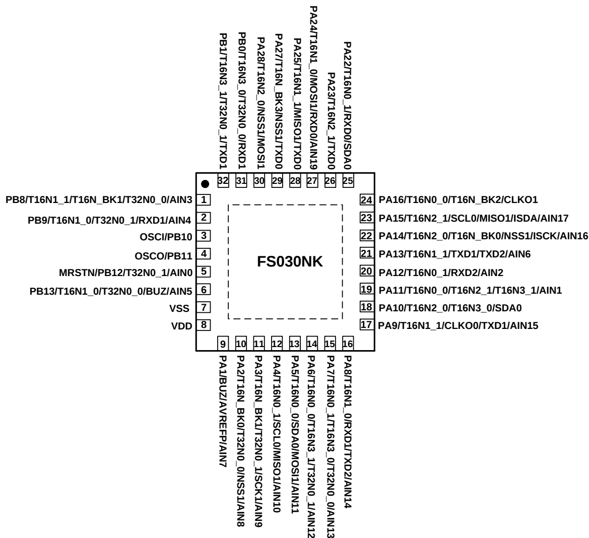
图 1-3 QFN32 封装顶视图(FS030NK)
