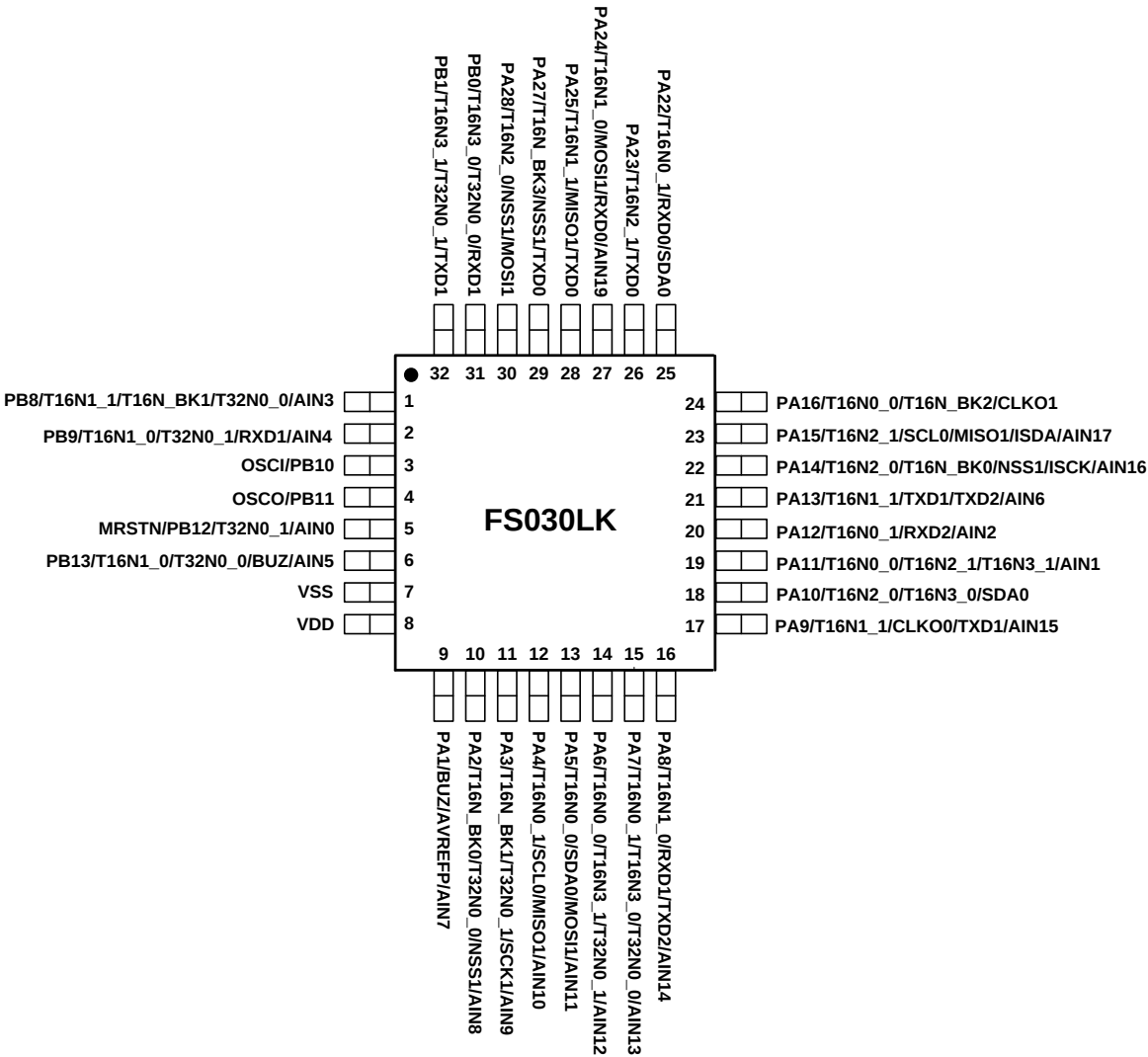
图 1-2 LQFP32 封装顶视图（FS030LK）
