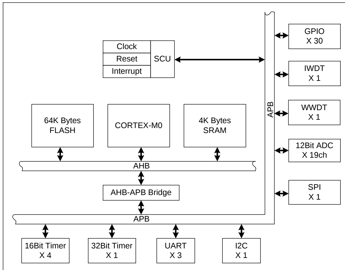
图 1-1 FS030 结构框图
