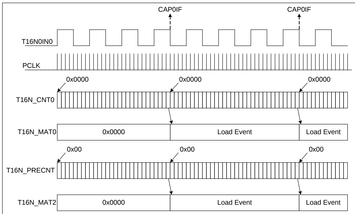
图 5-3 T16N0 捕捉功能示意图
