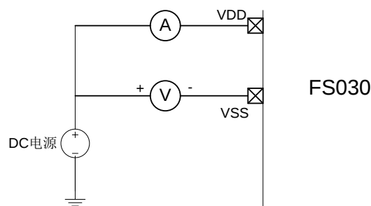
芯片功耗测量连接示意图
