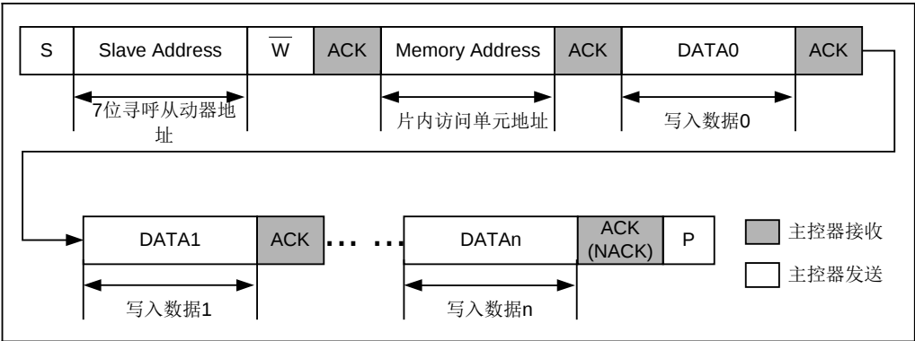
图 5-34 I2C 主控器写入从动器数据示意图
