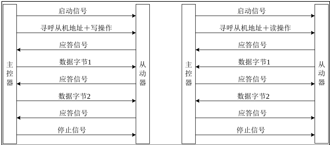
图 5-33 I2C 总线通讯协议示意图
