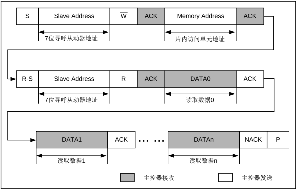
图 5-35 I2C 主控器读取从动器数据示意图
